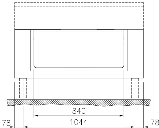
Zij aanzicht
